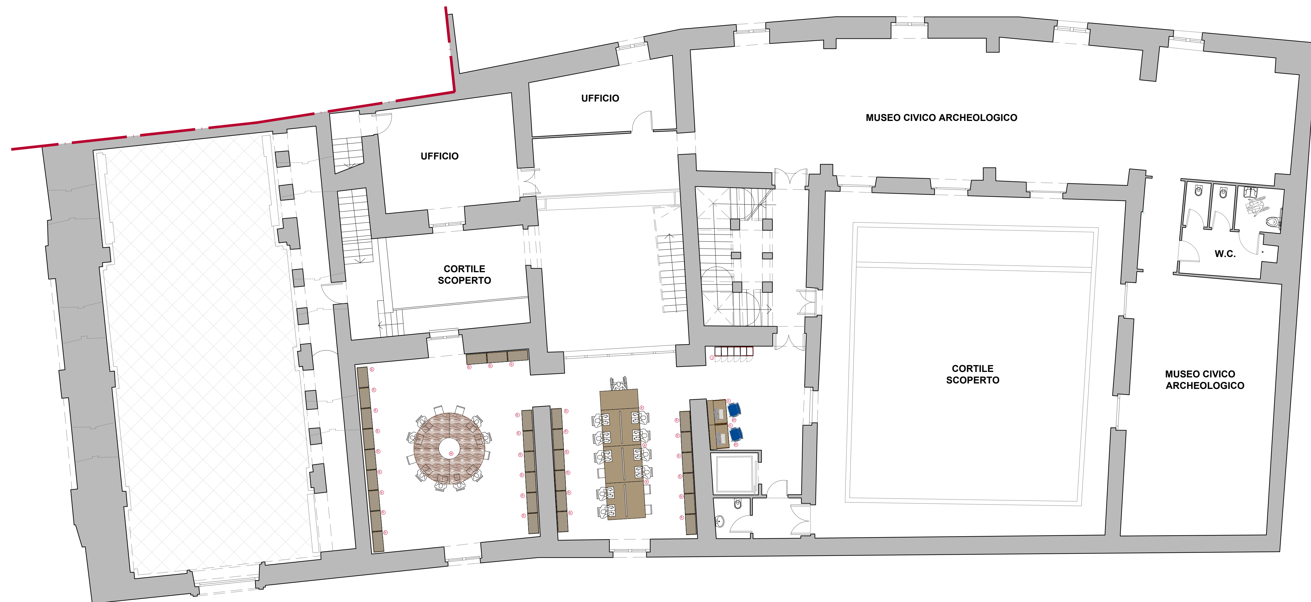
Pianta piano secondo scala 1:100
