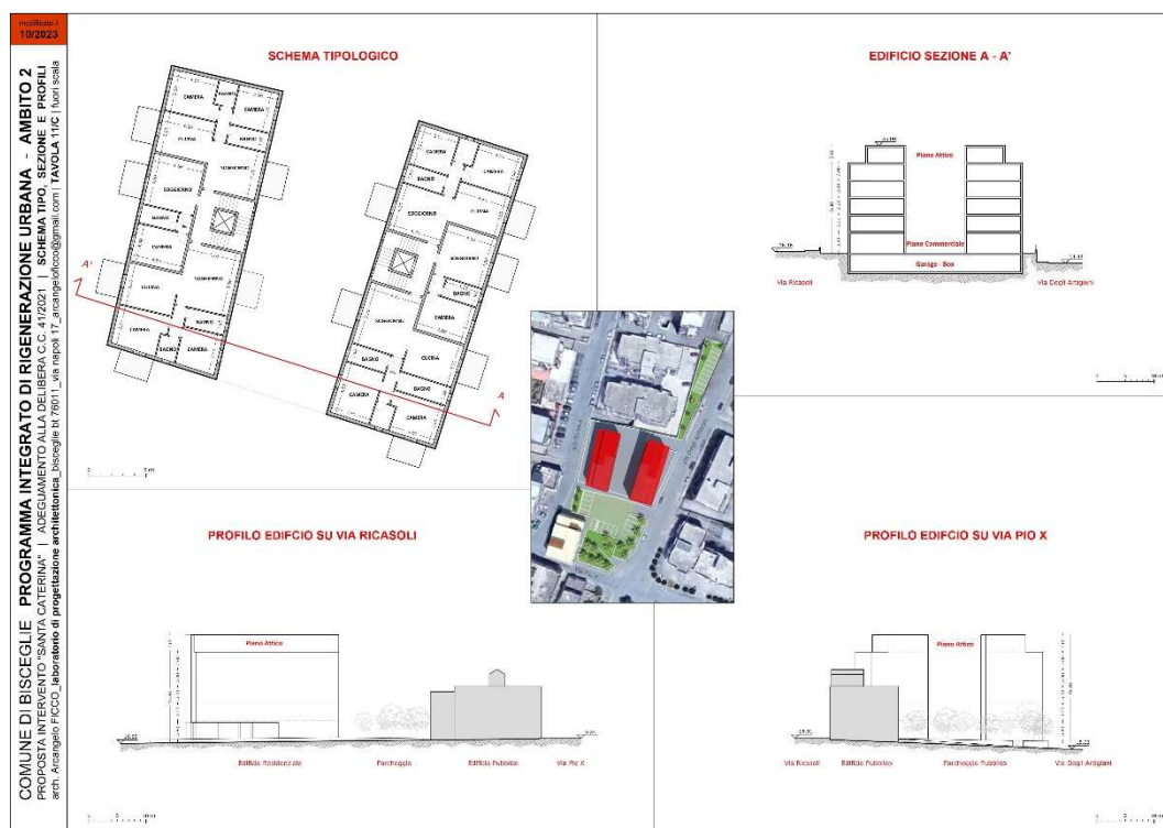
TAVOLA 11/C - schema tipologico, sezione e profili
