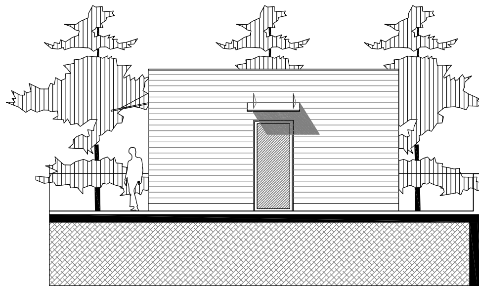
PROSPETTO OVEST (facciata laterale - ingresso servizi wc)
