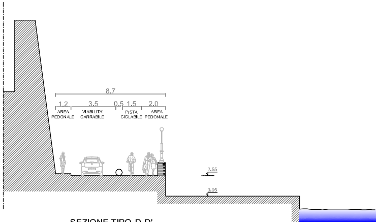
SEZIONE TIPO D-D'
