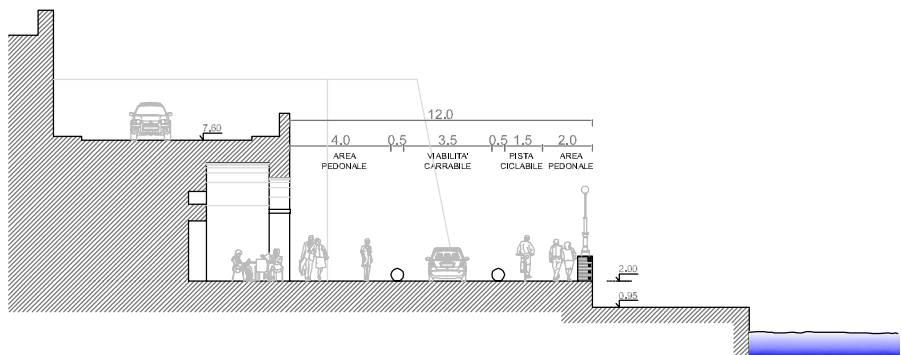
SEZIONE TIPO B-B'
