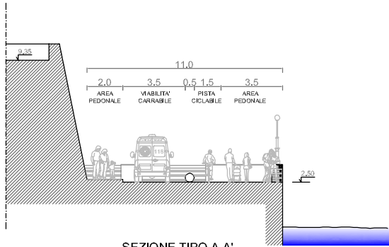
SEZIONE TIPO A-A'
