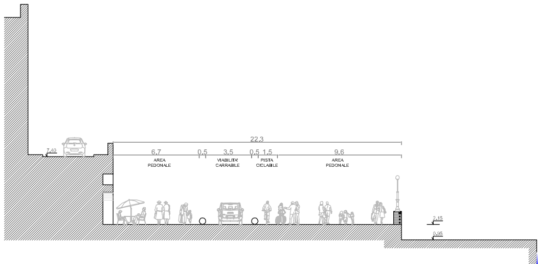
SEZIONE TIPO C-C'
