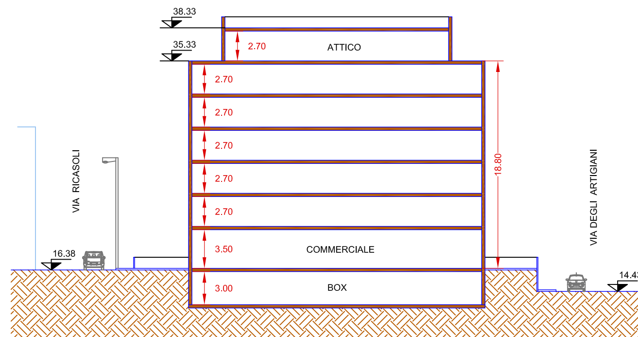
SEZIONE A-A
