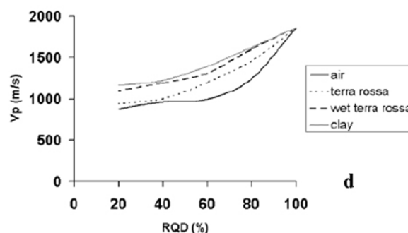
Fig. 30 - Correlazione velocità sismica/RQD per le calcareniti (Leucci, De Giorgi – 2003)
