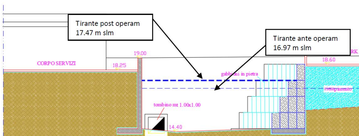
Fig. 19 – Sezione post operam con indicazione dei tiranti idrici
