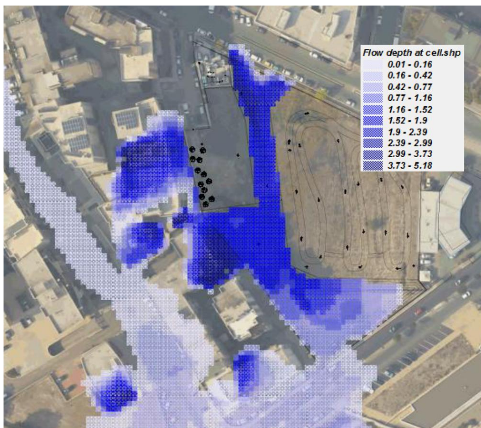
Fig. 20 – Tiranti idraulici post operam per tr 200 anni
