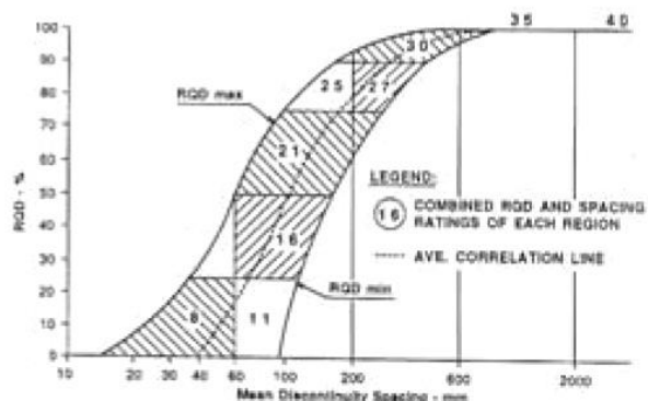
Fig. 28 – Correlazioni tra c_{amm}/c_{lab} e n° fratture (Manev ed Avramova-Tacheva-70) e tra RQD e discontinuità (Bieniawski)
