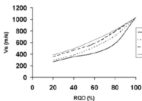
Fig. 30 - Correlazione velocità sismica/RQD per le calcareniti (Leucci, De Giorgi – 2003)
