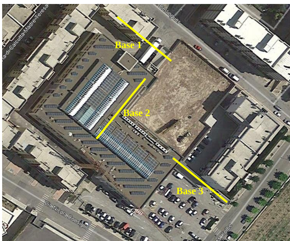
Fig. 24 – Ubicazione indagine sismica
