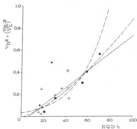
Fig. 29 – Correlazione tra V e RQD (Budetta e a. 01 - Zezza 75)
