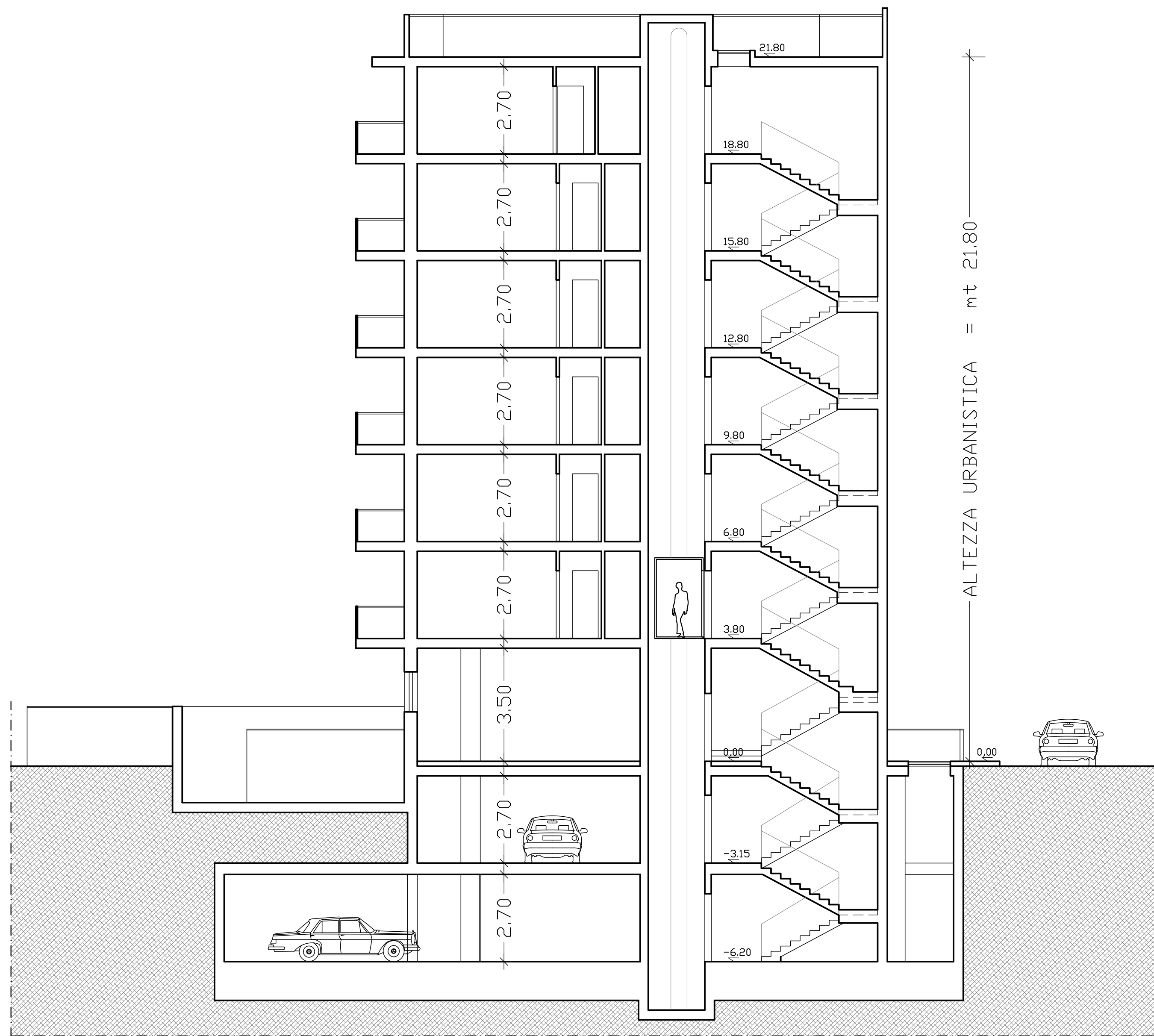
SEZIONE X - X
