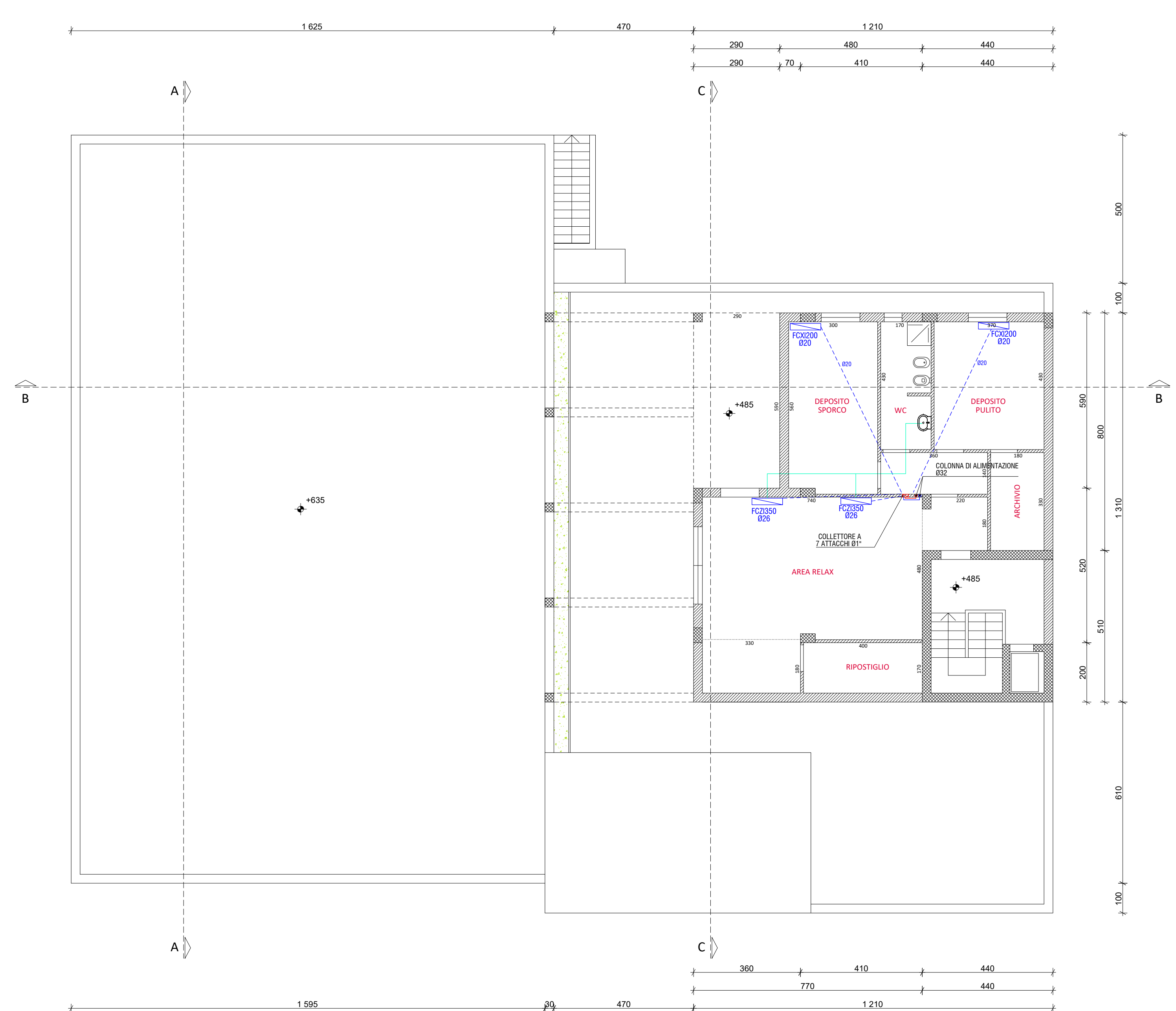
IMPIANTO TERMICO VENTILCONVETTORI - piano primo scala 1:100
