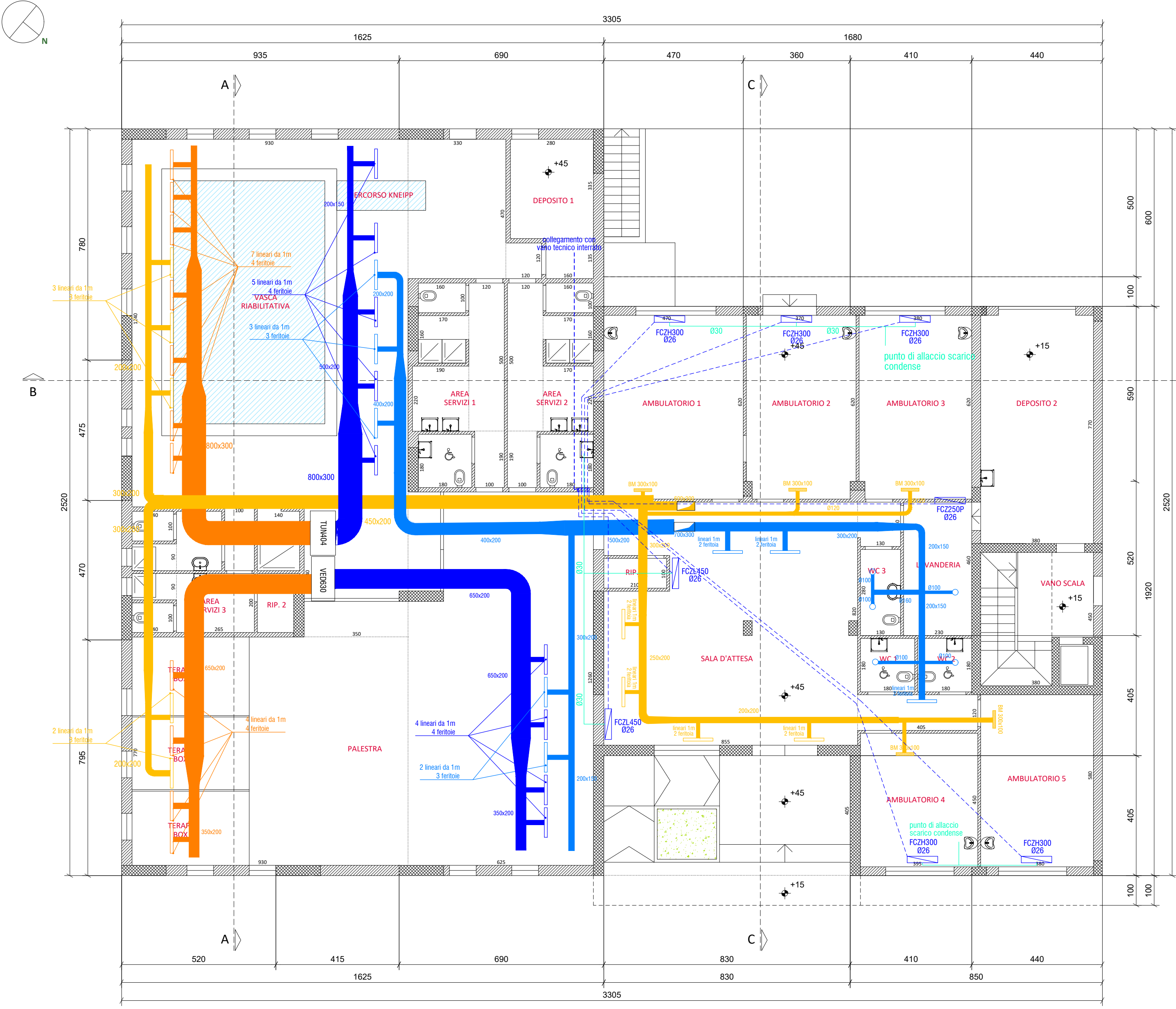
IMPIANTO TERMICO VENTILCONVETTORI - piano terra scala 1:100
