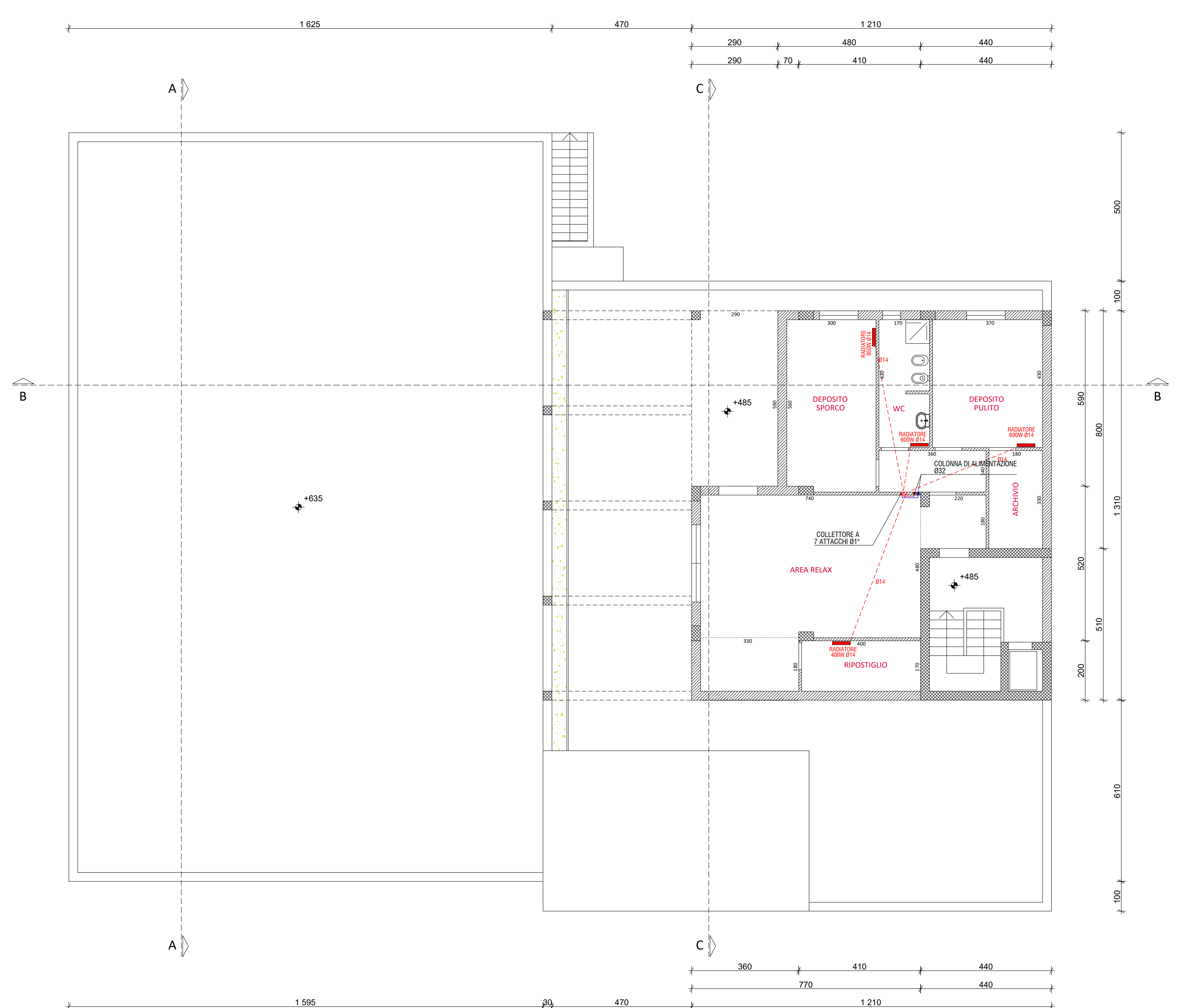
IMPIANTO TERMICO RADIATORI - piano primo scala 1:100
