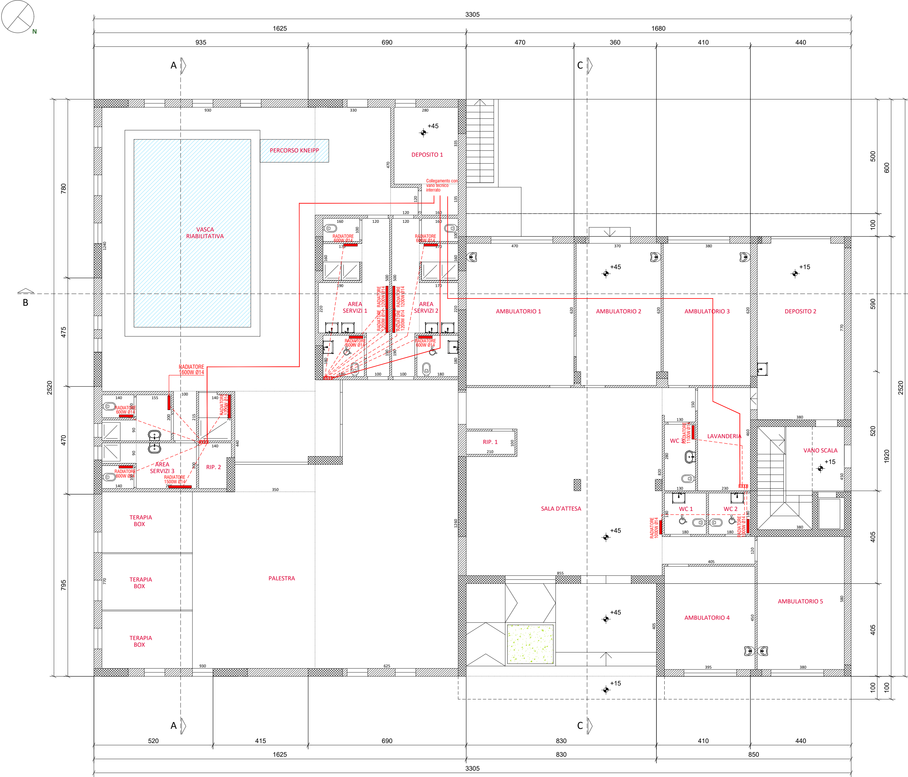
IMPIANTO TERMICO RADIATORI - piano terra scala 1:100
