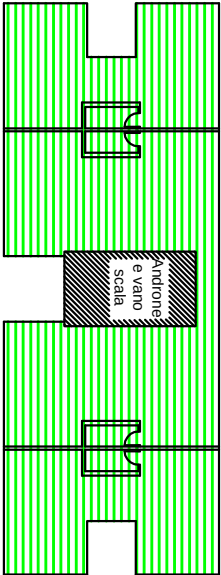
PIANTA PIANO TERRA Locali commerciali h :3.50 Superficie coperta : 497.81 mq Volume di progetto : [497.81 * (3.50 + 0.3)] = 1891.68 mc
