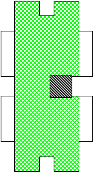
PIANTA PIANO TIPO Sup.coperta: 510.4 mq h: 15.00 m Volume: 7656 mc
