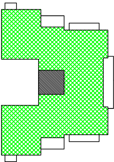
PIANTA PIANO TIPO Sup.coperta: 515.93 mq h: 15.00 m Volume: 7738.95 mc
