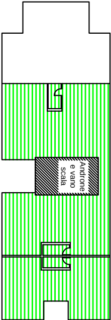
PIANTA PIANO TERRA Locali commerciali h :3.50 Superficie coperta : 415.49 mq Volume di progetto : [415.49 * (3.50 + 0.3)] = 1578.86 mc
