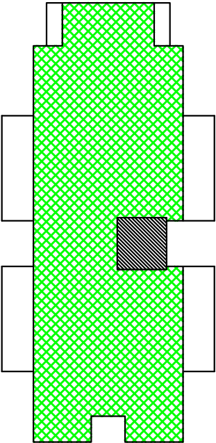
PIANTA PIANO TIPO Sup.coperta: 557,4 mq h: 15,00 m Volume: 8361 mc
