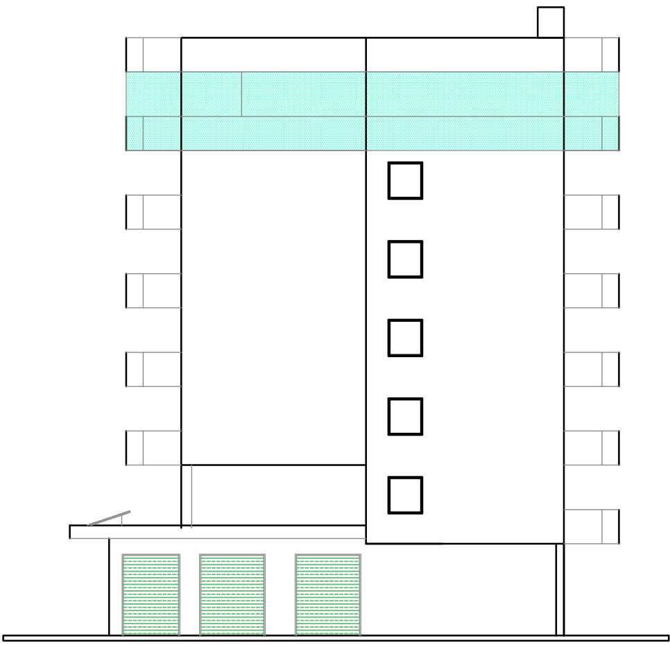
PROSPETTO EST
