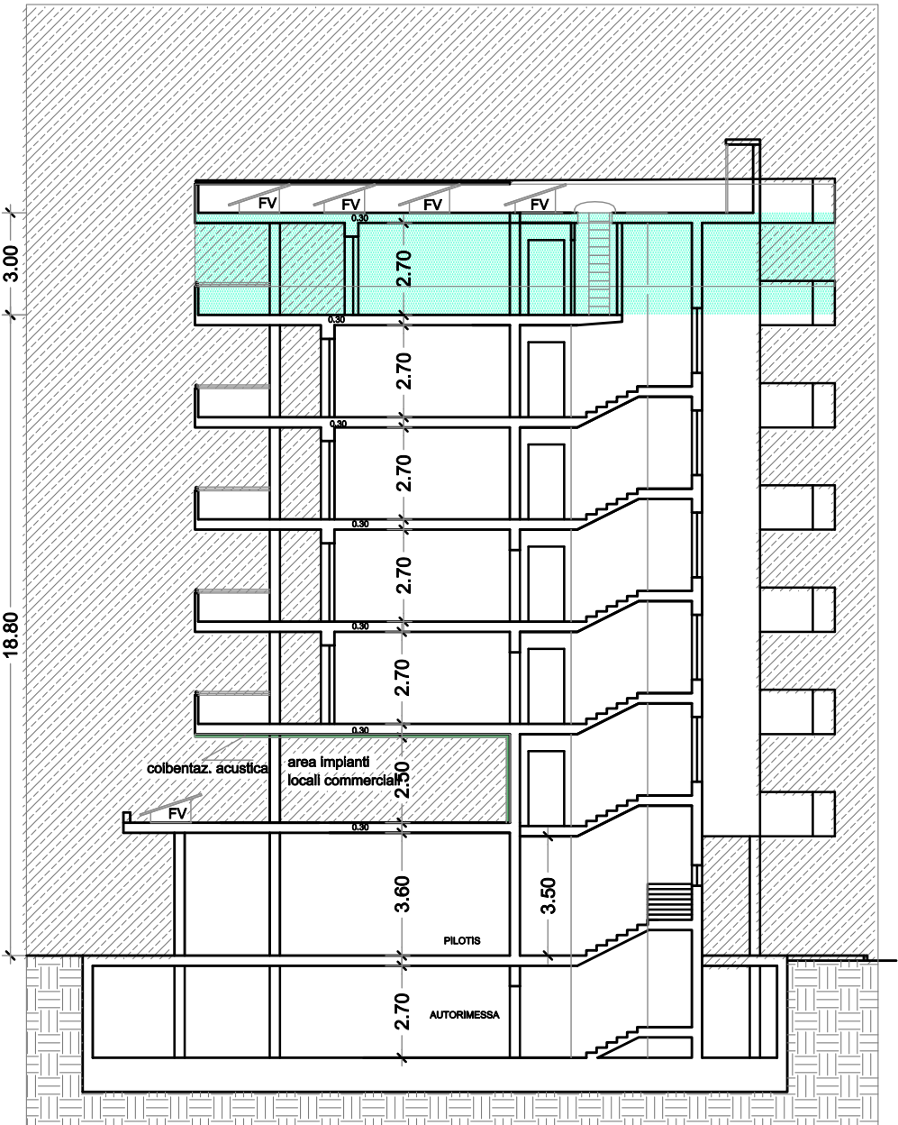
SEZIONE Y - Y
